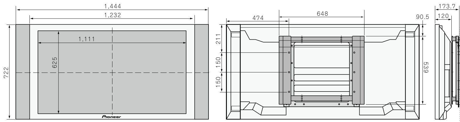
垂直固定金具使用時 (RA-PDPV50+WA-PD02)
